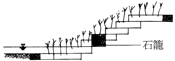
圖十一 石籠護岸
