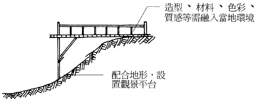
圖三 平台設置示意圖
