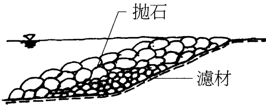
圖十 拋石護岸
