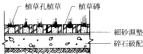
圖一 植草磚鋪面剖面圖
