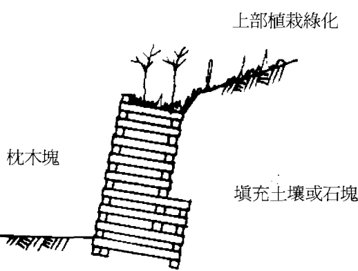
圖六 木材邊坡
