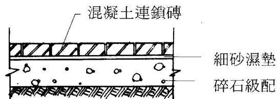
圖二 混凝土連鎖鋪面剖面圖
